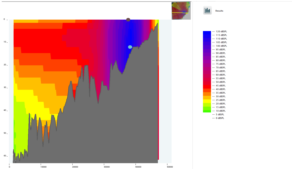
Figuri 9-2. Esimerkki ruoppauksesta aiheutuvan melun leviämisestä vertikaalisesti (syvyysuuntaisesti).
